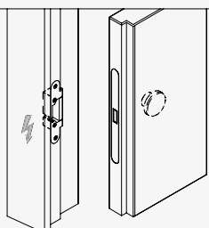
Serratura contact (incontro magnetico) con leva tira porta a incasso LARGE
