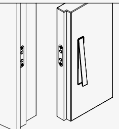
Serratura contact (incontro magnetico) con leva tira porta a incasso SLIM
